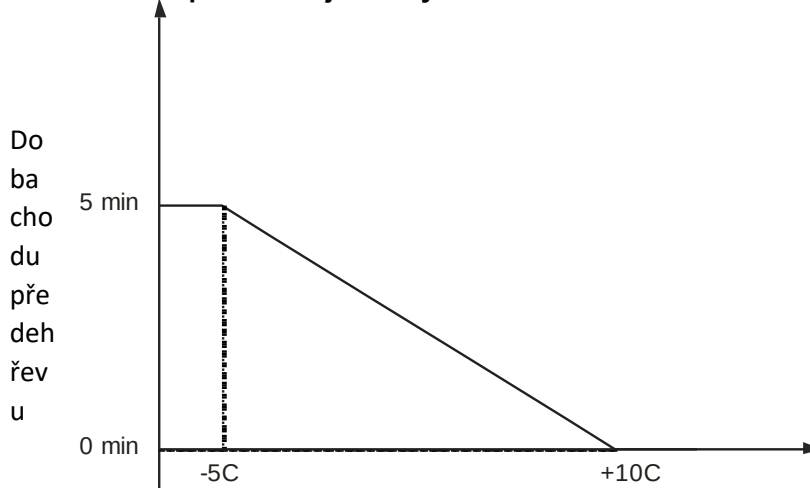
Křivka přehřátí jednotky:
