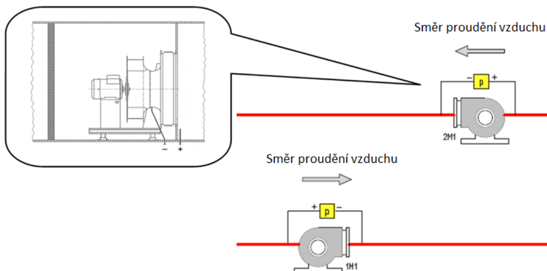
Obr. 3.2 Tovární instalace v zařízení
