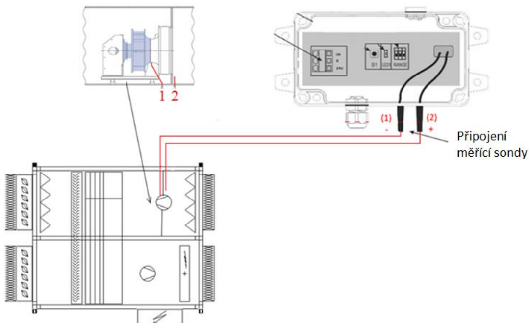
Obr. 3.2 Tovární instalace v zařízení
