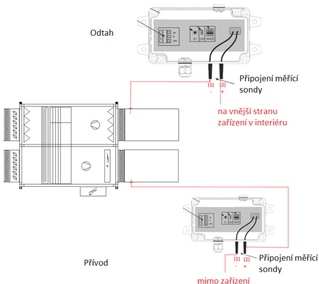
Obr. 2.1 Instalace měřicích hadiček v potrubí
